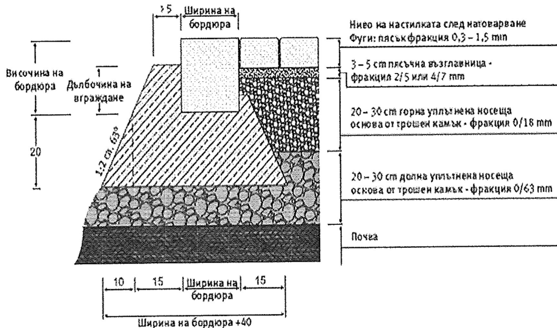
Бетоново легло
